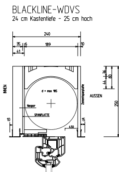
Mauerwerk 24 cm
