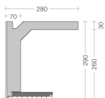
Halbschale 28 cm
