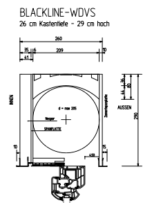
Mauerwerk 26 cm
