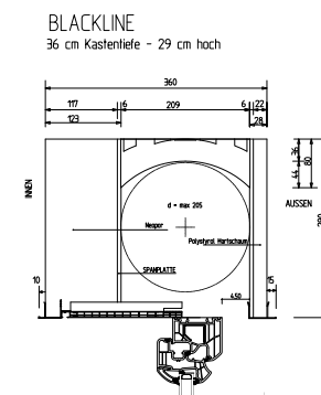
Mauerwerk 36 cm
