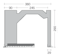
Mauerwerk 36 cm
