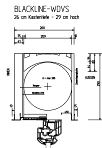
Mauerwerk 26 cm
