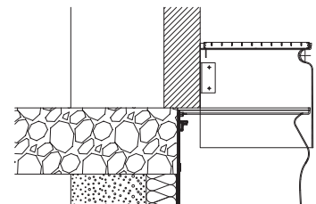
Lichtschacht MEAMULTINORM mit verkürztem Aufsatz
