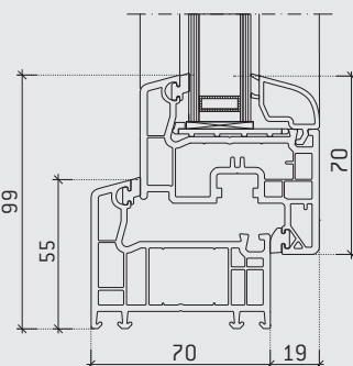
Querschnitt MEALON Komfort
