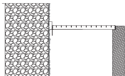
Standard-Rosttiefe, Wandabstand 3,0 cm
