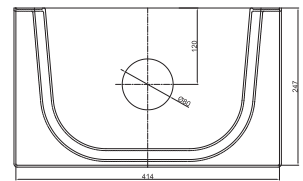
Lüftungsschacht mit Boden und Entwässerungsöffnung Ø 80 mm
