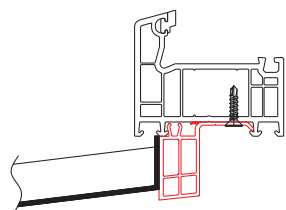
Fensterbankanschluss, Einbaubeispiel
