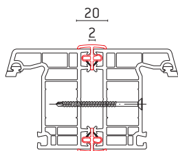
Kopplung, Einbaubeispiel (Abmessungen in mm)
