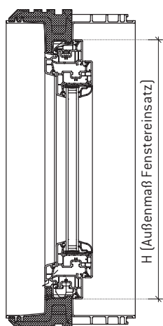
Querschnitt Zarge MEALUXIT mit Dreh-Kipp Einsatz
