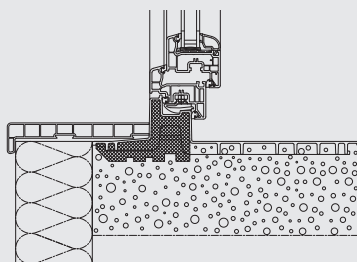
Querschnitt Zarge MEALUXIT mit Perimeter-Abdeckrahmen MEAFRAME
