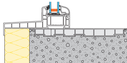
Ausführung B: betonierte Wände
