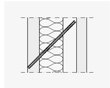
Einbau Schöck Isolink® Typ C-ED
