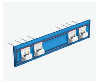
Schöck Tronsole® Typ T für negative Fertigung
