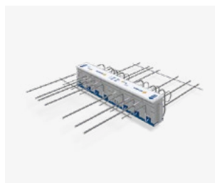
Schöck Isokorb® XT Typ K-BH
