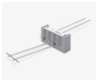
Schöck Isokorb® RT Typ Q-P positive Querkraft
