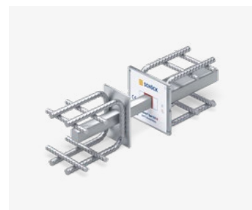
Schöck Stacon® Typ SLD-Q (längs- und querverschieblich)
