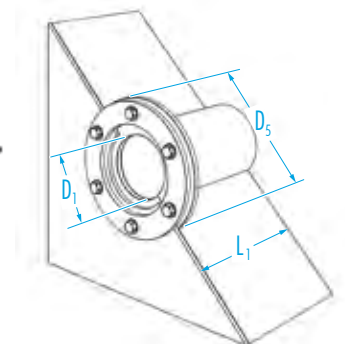
Variante: Curaflex® 4005/U als Sohlendurchführung
