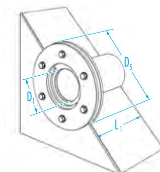
Variante: Curaflex® 4006/U als Sohlendurchführung
