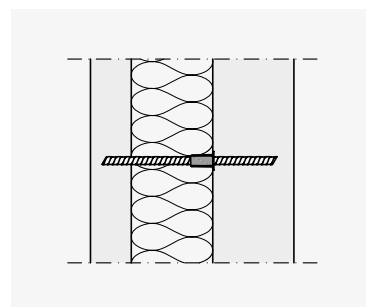
Einbau Schöck Isolink® Typ C-SH
