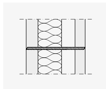
Einbau Schöck Isolink® Typ C-EH
