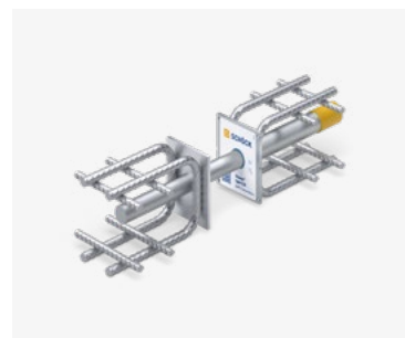
Schöck Stacon® Typ SLD
